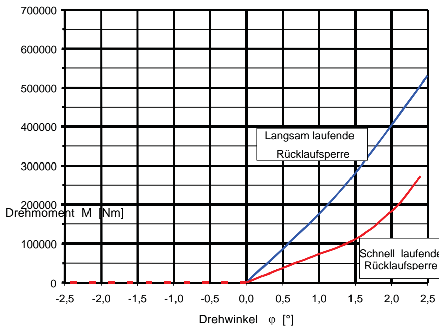
Bild 1: Drehfederkennlinien von langsam- und schnellaufenden Rücklaufsperrern
