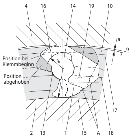
4: Klemmstück im Käfig der neuen Generation für Abhebung X
