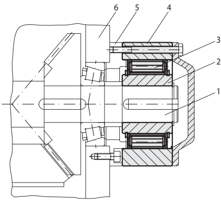
2: Kegelstirnrad-Getriebe mit Anbaufreilauf als Rücklaufsperr
