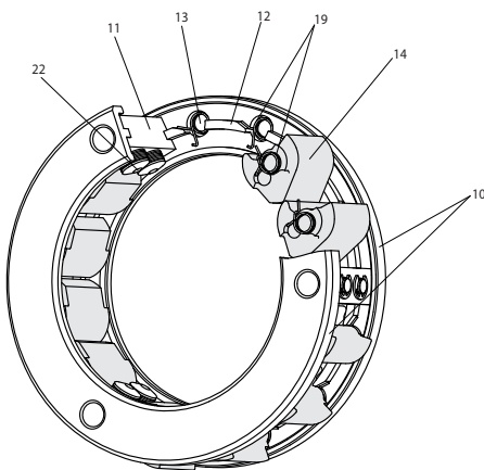
3: Perspektivische Darstellung des Freilaufkäfigs
